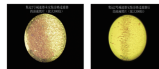
油液过滤前，后在300倍显微镜下照片
